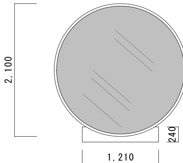
背面図
